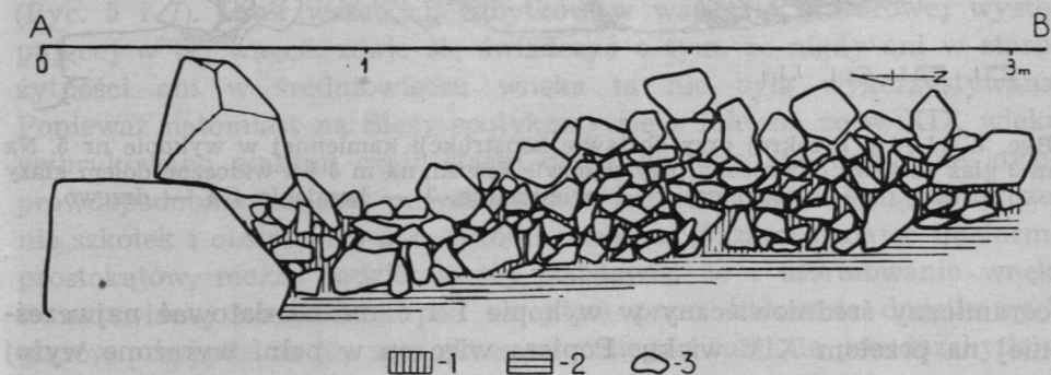
Ryc. 6. Ślęża. Przekrój przez konstrukcję na wykopie nr 3. Widoczna warstwa nałożonych kamieni, a na m 0. — 1 gład obstawy. 1 — próchnica, 2 — zwietrzelina, 3 — kamienie.
