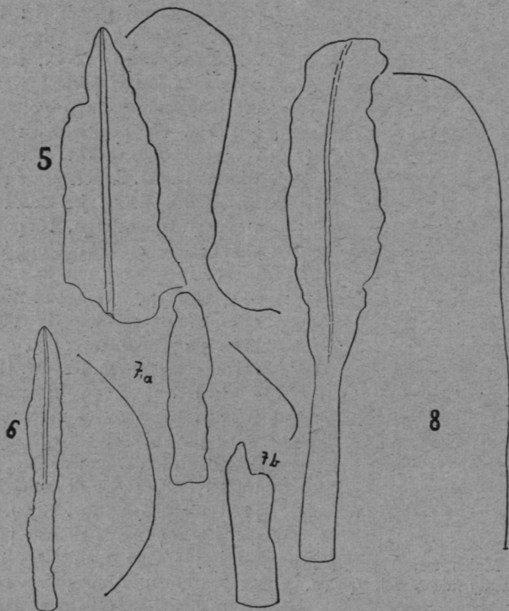
Rys 5—8. Malkowice, pow. Pińczów. Żelazne groty oszczepów, \frac{1}{3} w. n.
